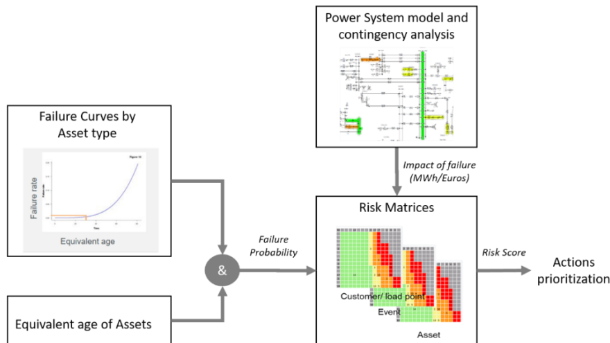
Figure 2.12 : Prise de décision future basée sur le risque pour la gestion du déclassement ou du remplacement des équipements
