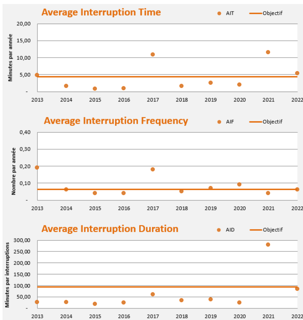
Figure 4.2 : Evolution des indicateurs de fiabilité sur les 10 dernières années
